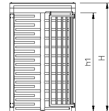
Kentaur – FTS E01, ohrazen z boku ocelovými tyčemi.
