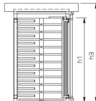
Kentaur – FTS E03, L04, ochrana před vlivem prostředí – stříška s fascií a odpadem
