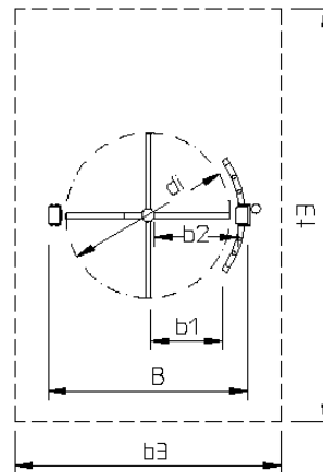
Kentaur – FTS E03, L04, ochrana před vlivem prostředí – stříška s fascií a odpadem
